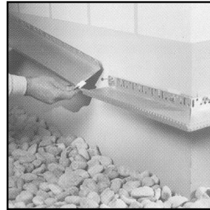
Ansetzen und Befestigen (Bohren) der Sockelabschlussleisten, wobei Sockelabschlussleistenstöße mit Sockelabschlussleistenverbindern fachgerecht überbrückt werden. Niveauunterschiede des Untergrundes mit Unterlegscheiben ausgleichen.
